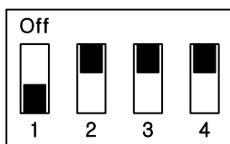
② Bus Topology 종단 사용 (100 Ohm)
