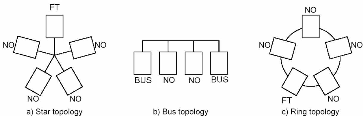
다른 Network Topology에 따른 종단 형태
